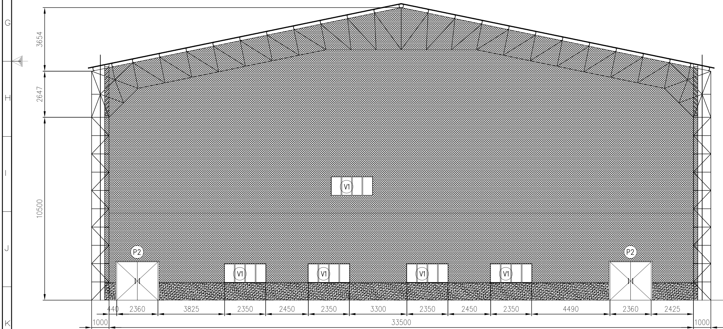
VISTA E - E (Fachada Oeste)
